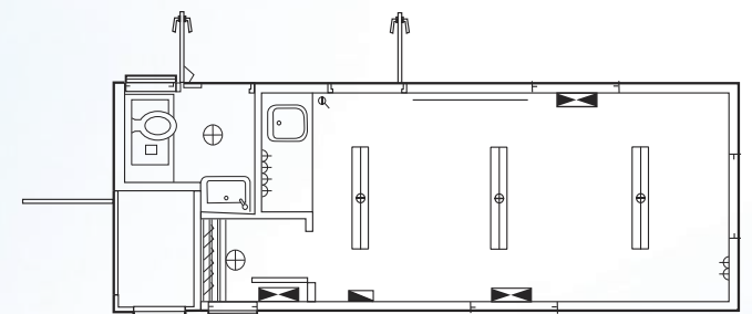
WelGen 700
